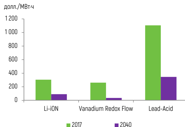
Рисунок 1.24 – Прогноз сокращения приведенной стоимости хранения (LCOS) электроэнергии до 2040 г. для различных технологий, долл./МВт·ч
