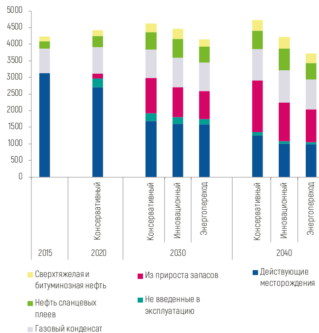
Рисунок 2.36- Добыча нефти по видам, по сценариям
