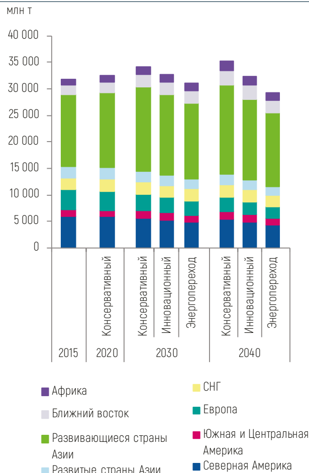
Рисунок 2.65 - Динамика выбросов CO 2 по региону мира 37
