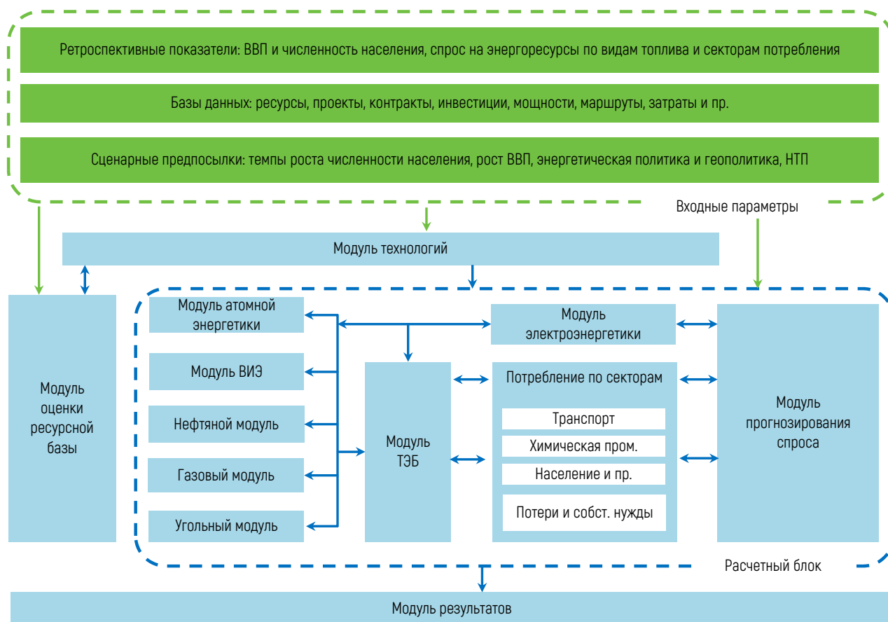
Рисунок 1.8 – Схема моделей прогнозирования мировой энергетики комплекса SCANNER
