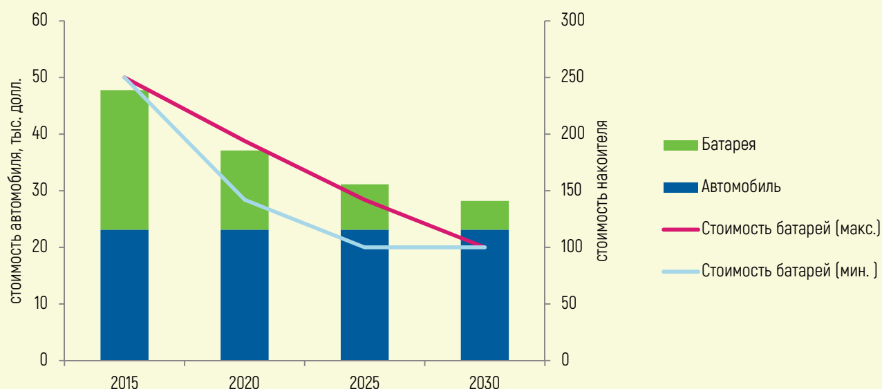
Рисунок 1.25 – Структура затрат в до-налоговой стоимости электромобиля в США и прогнозные затраты на производство батарей
