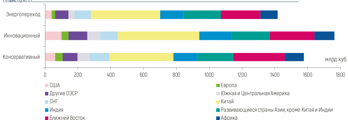
Рисунок 2.48- Сценарный прогноз прироста спроса на газ в период с 2015 по 2040 гг. по регионам и крупнейшим странам мира, млрд куб. м
