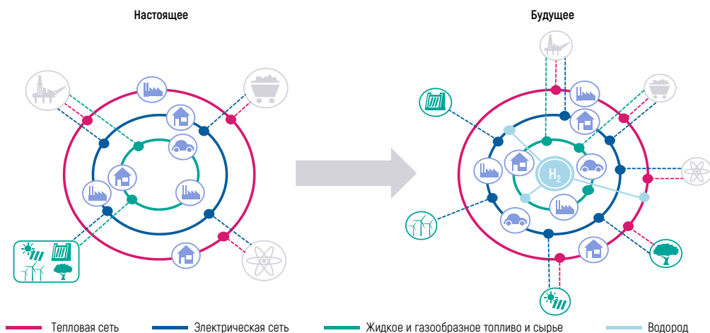
Рисунок 1.26 – Место водорода как нового глобального энергоносителя в интегрированном энергетическом комплексе
