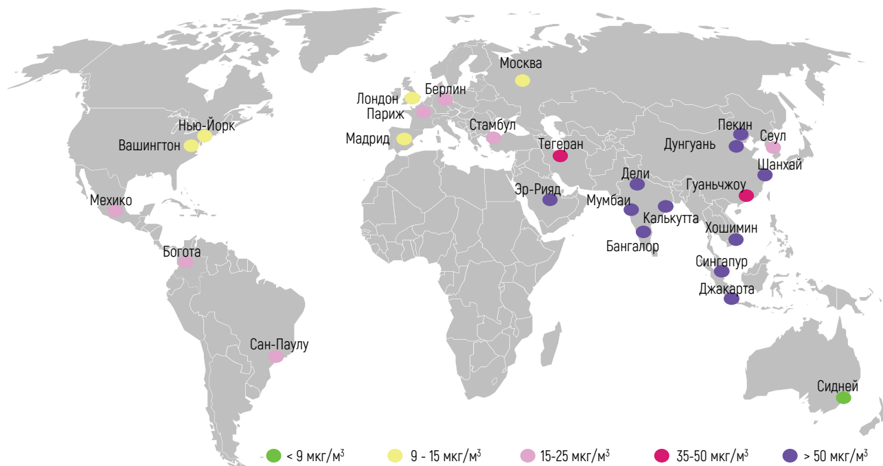
Рисунок 1.12 – Индекс качества воздуха 2018
