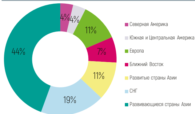
Рисунок 2.21 - Доли строящихся энергоблоков по регионам мира по состоянию на июнь 2019 г.
