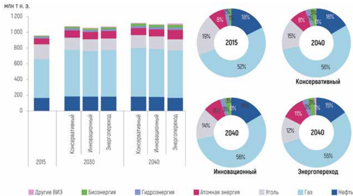
Рисунок П3.7 - Потребление первичной энергии по видам топлив и его структура по сценариям в СНГ
