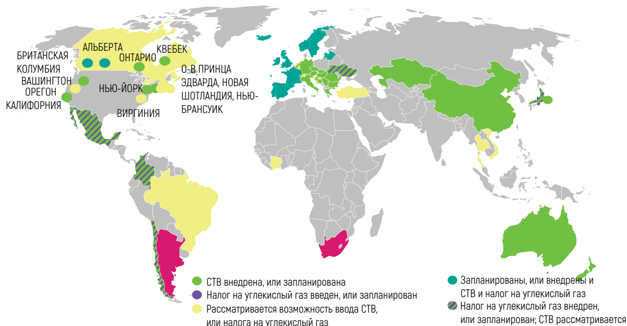
Рисунок 1.11 – Статус национальных систем торговли выбросами (СТВ) и систем углеродных сборов в мире по состоянию на 2018 г.
