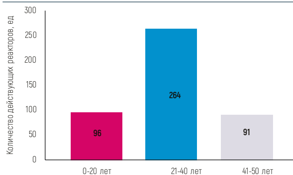
Рисунок 2.22 - Возраст действующих в мире энергоблоков по состоянию на июнь 2019 г.
