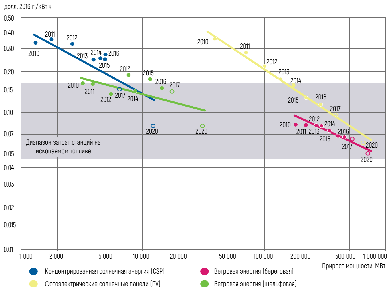
Рисунок 1.20 – Кривые обучения по полным приведенным затратам для основных технологий ВИЭ, 2010-2020 гг.
