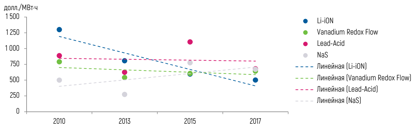
Рисунок 1.23 – Приведенная стоимость хранения электроэнергии для различных технологий (системы в сборе)
